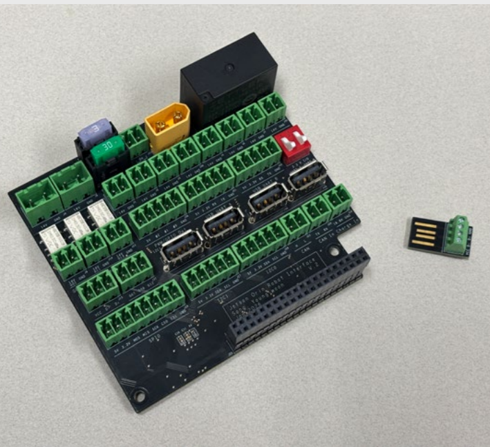
▲ Standardised Robot Interface Board for Jetson Orin-Based Systems (Jan 2026) Standardisiertes Roboter-Interface-Board für Jetson Orin-Systeme (Jan. 2026)
