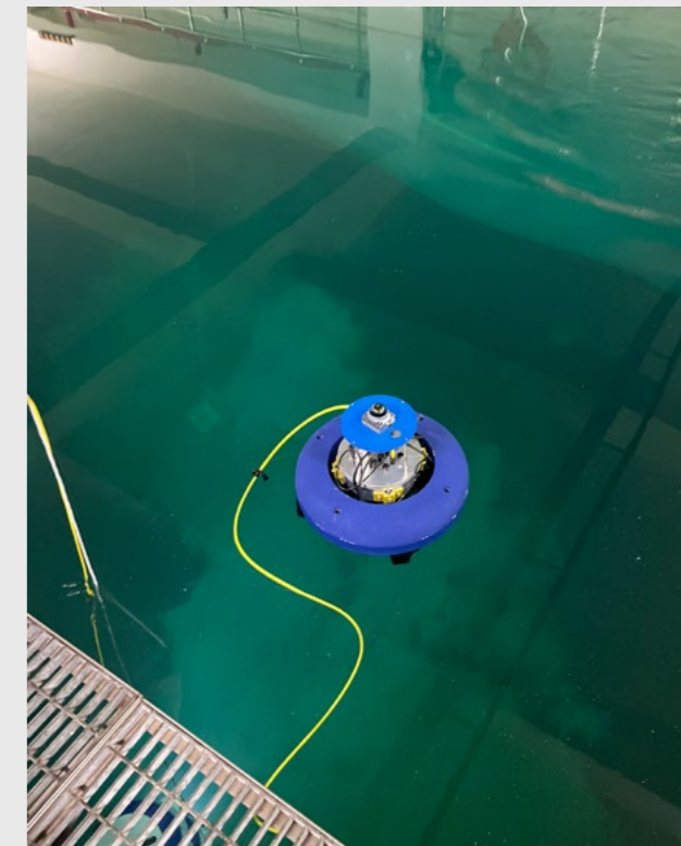
▼ Autonomous Surface Vehicle (ASV) Using the Developed Robot Interface Board (Sep 2025) Autonomes Oberflächenfahrzeug (ASV) mit dem entwickelten Roboter-Interface-Board (Sep. 2025)
